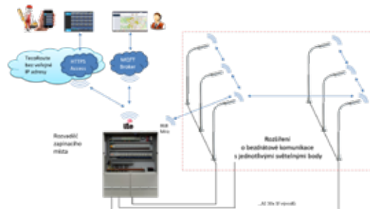
Obr. Koncept bezdrátové komunikace zapínacího místa veřejného osvětlení na nadřazený dispečink, komunikace se servisním personálem a komunikace s každým podřízeným světelným bodem. Komunikační a řídicí centrálou je tu nový Foxtrot 2 a přes jeho síť v pásmu 868 MHz lze připojovat i další senzory a přirozeně tak rozšiřovat internet věcí (IoT).
